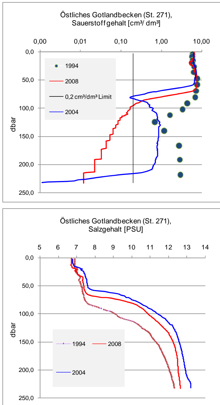
Abb. 16: (a) Vertikalprofil des Sauerstoffgehaltes im Gotlandtieft jeweils im August 1994, 2004 und 2008, d.h. nach dem Salzwassereinbruch vom Frühjahr 1993, dem vom Sommer 2003 und während der anhaltenden Stagnation im Jahre 2008 sowie zur Orientierung, die suboptimalen Bedingungen mit 0,2 \text{ cm}^3/\text{dm}^3 und (b) die dazugehörigen Salzgehaltsprofile.
