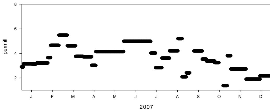
Abb. 11: Isotopie des Stickstoffs (permil delta ^{15}\text{N} ) im Fallenmaterial im Jahr 2007.
