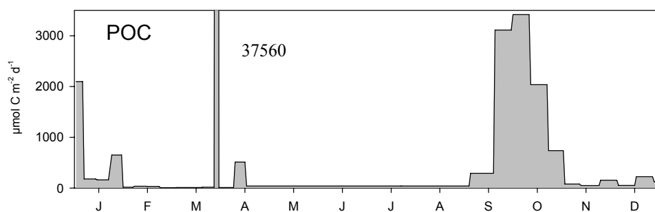
Abb. 10 Tägliche Sedimentationsraten von partikulärem organischem Kohlenstoff im Sedimentationshorizont 140 m auf der Station 271 im Jahre 2001
